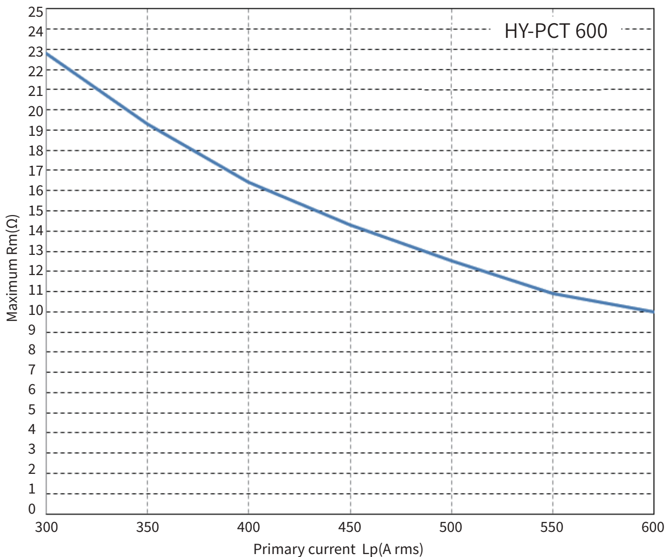
HY-PCT 600 负载电阻与测量电流关系图 示例图
