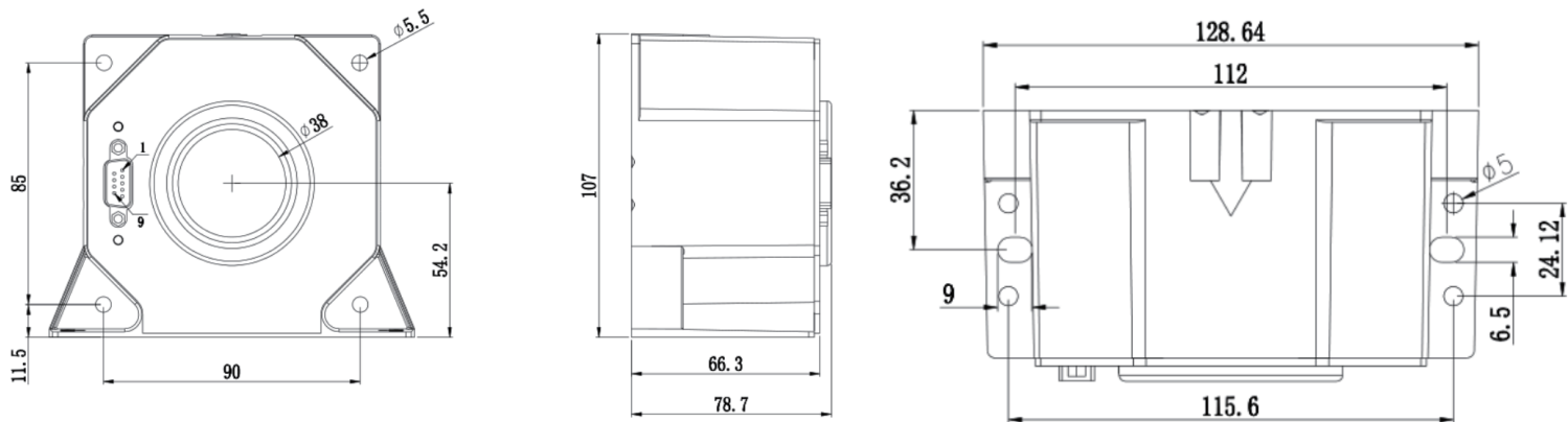
单位:毫米(mm) HY-PCT 1500尺寸示意图
