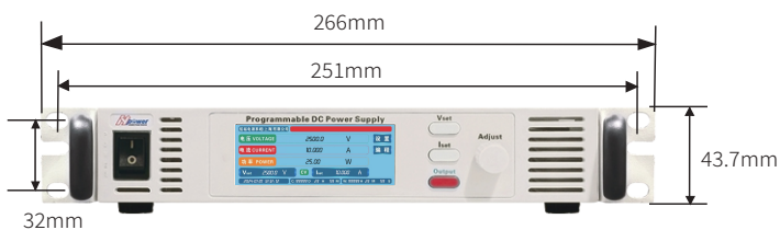
正视图
