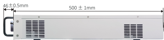
侧视图
