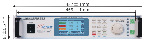
正视图
