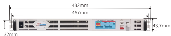
正视图
