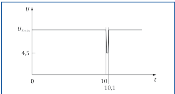
图7-12V电力系统短电压降
