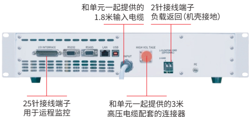
后视图
