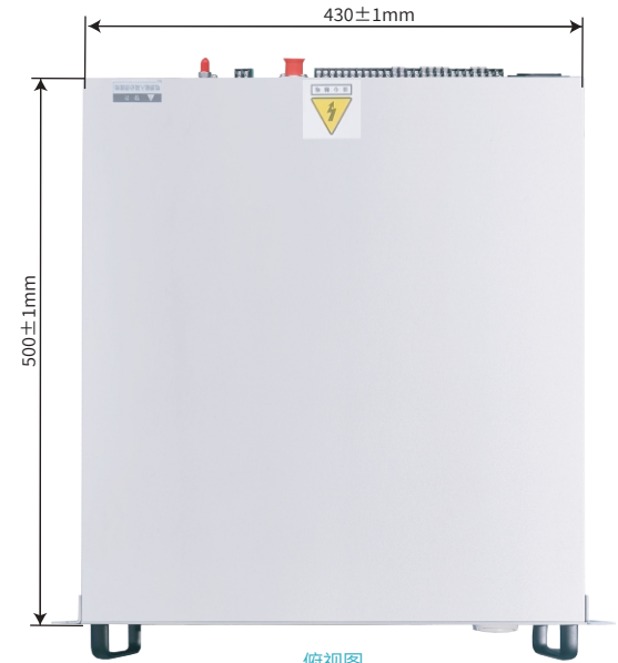
俯视图
