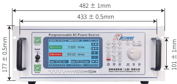
4U 433(W)*560(D)*177(H)mm
