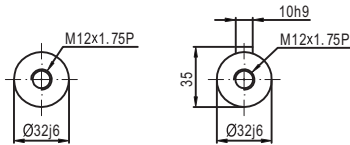
轴型式 S1 shaft 轴型式 S2 shaft
