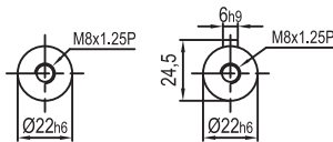
轴型式 S1 shaft
