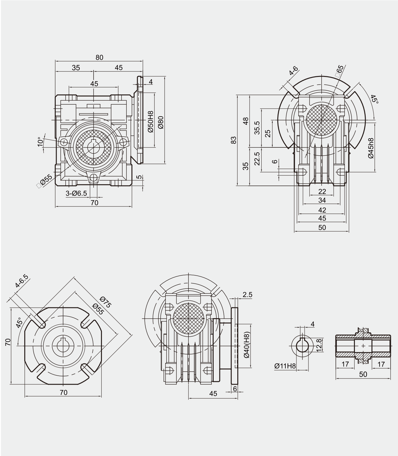
NMRV 025外形尺寸 / Outline Dimension
