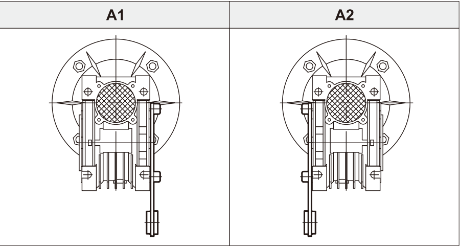
扭力臂 ( A ) 位置 / Torque arm (A) position
