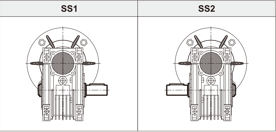
扭力臂 ( A ) 位置 / Torque arm (A) position
